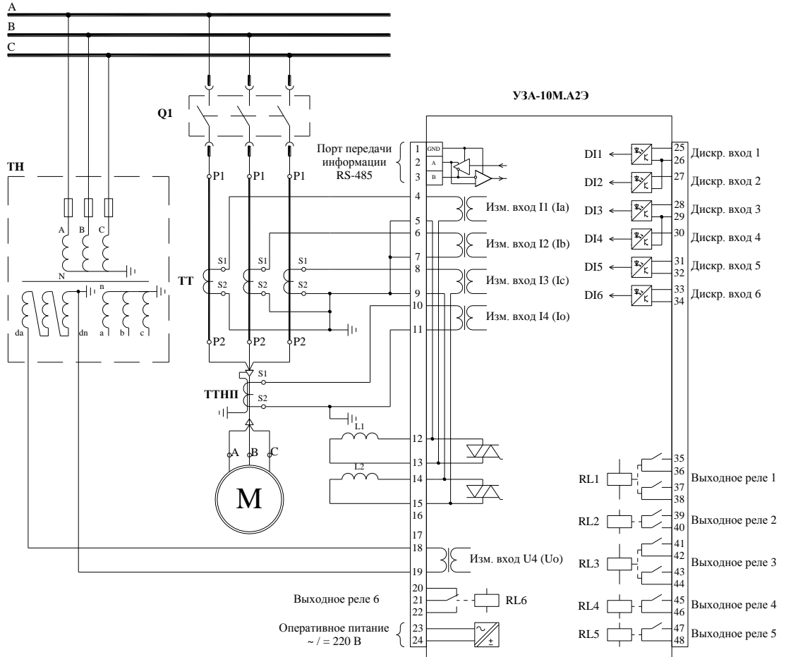
Рисунок 2. Схема подключения УЗА-10М.А2Э с выходом дещунтирования электромагнитов отключения.
