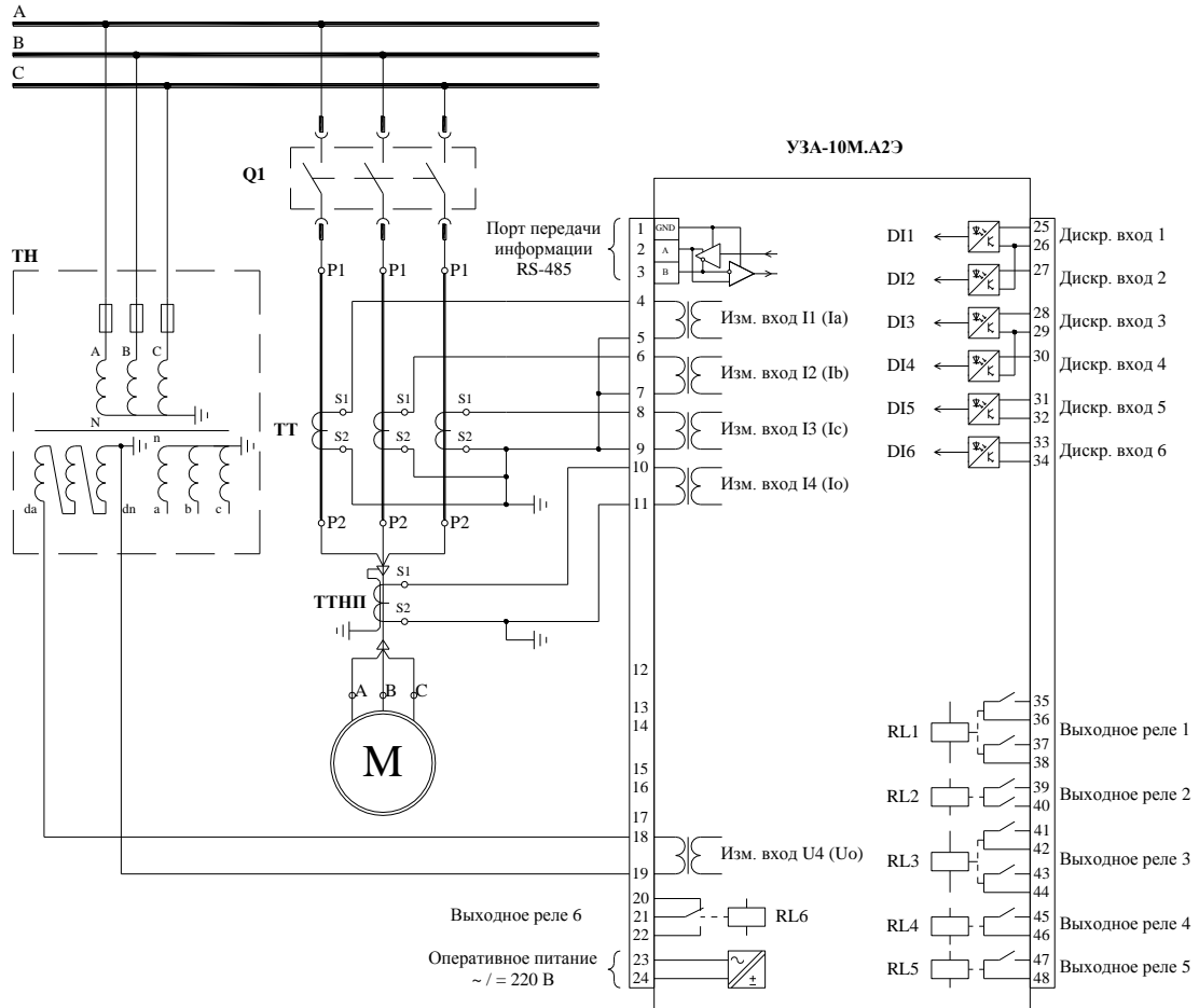
Рисунок 1. Схема подключения УЗА-10М.А2Э без выхода дещунтирования электромагнитов отключения
