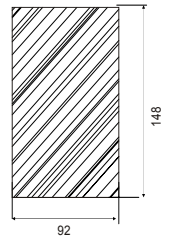
ВЫРЕЗАЕМОЕ ОТВЕРСТИЕ В ДВЕРИ РЕЛЕЙНОГО ШКАФА
